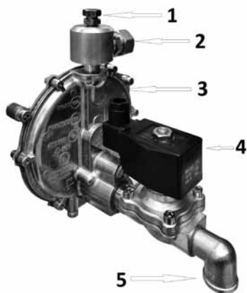
Рис. Внешний вид блока подключения топлива
